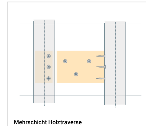
Mehrschicht Holztraverse
